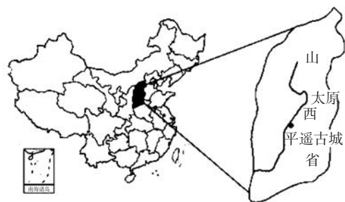
山西省在全国的位置 平遥古城在山西省的位置
