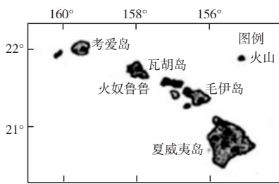
夏威夷群岛的位置和火山分布
