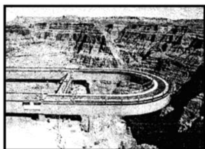
科罗拉多大峡谷局部
